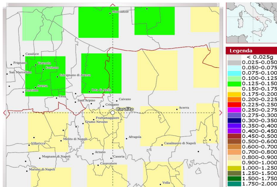
Mappa della pericolosità sismica del territorio comunale di Cardito (NA) dell'INGV con i range di valori delle ag nella legenda corrispondente
